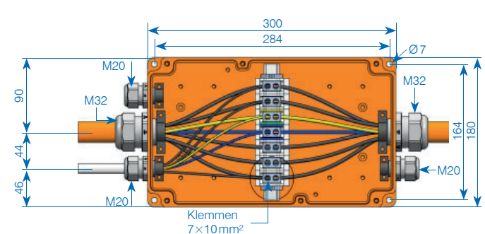
BFA 3018 – 300×180×100 mm / 7×10 mm 2 Art.-Nr.: 189887
