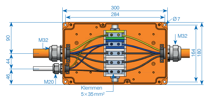
BFA 3018 – 300×180×100 mm / 5×35 mm 2 Art.-Nr.: 189886
